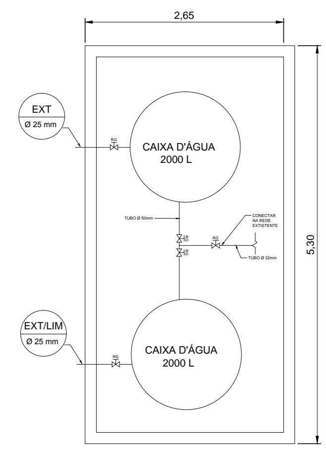
PLANTA DE COBERTURA - ÁGUA FRIA ESC.: 1/50
