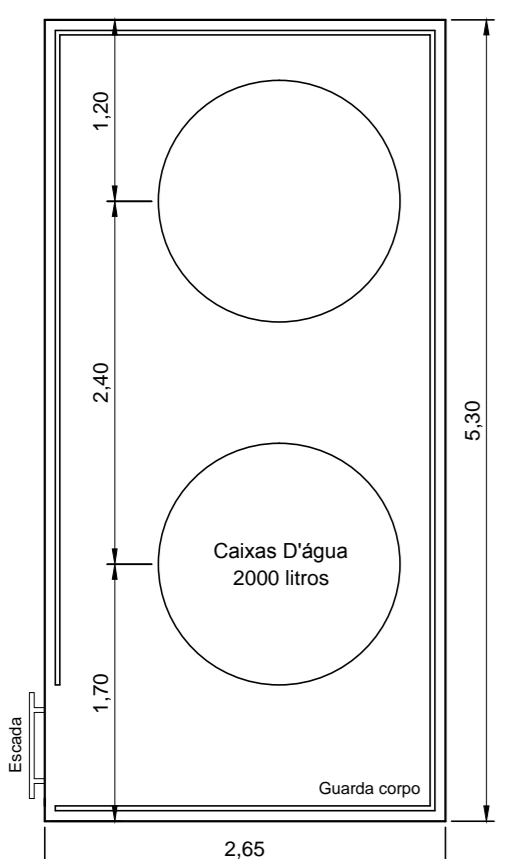
PLANTA BAIXA - NÍVEL CAIXAS ESC.: 1/50
