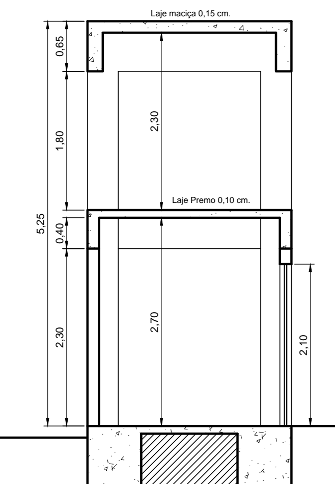
CORTE TRANSVERSAL ESC.: 1/50
