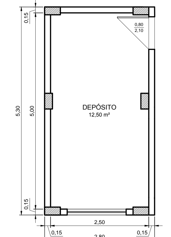
PLANTA BAIXA - TÉRREO ESC.: 1/50
